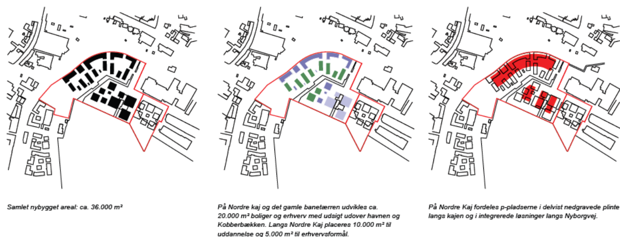
Figur 5. Udviklingsplan for Nordre Kaj. Venstre: sort angiver nye bygninger, midt: fordeling af erhverv, bolig og uddannelse. Højre illustrerer fordeling af parkeringspladser.
